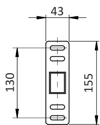
Rozměry uchycovací plotny držáků.
