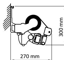
Montáž na stěnu
