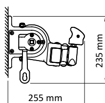
Montáž na stěnu
