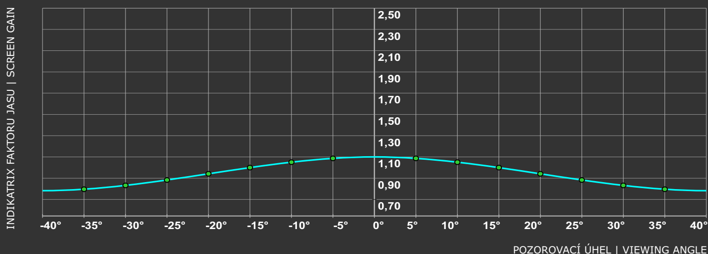
FAKTOR JASU MĚŘEN DLE DIN 19045 | GAIN ACCORDING TO DIN 19045
